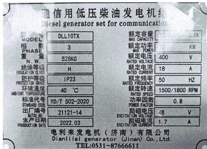
DLL10TX（10kW）
